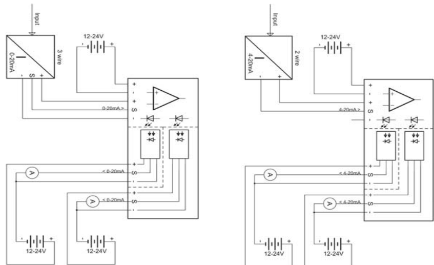
Primjer spajanja senzora sa dvije i tri žice
